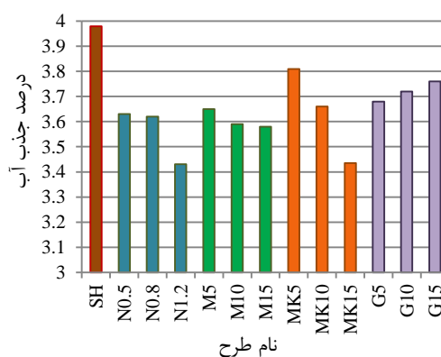
شکل ۷: درصد جذب آب مربوط به کلیه طرح‌ها
